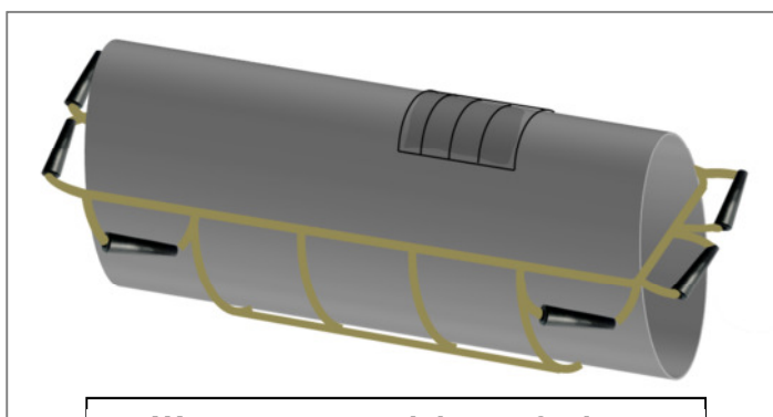
Warmwasserspeicher aufgelegt und Tragenetz angezogen
